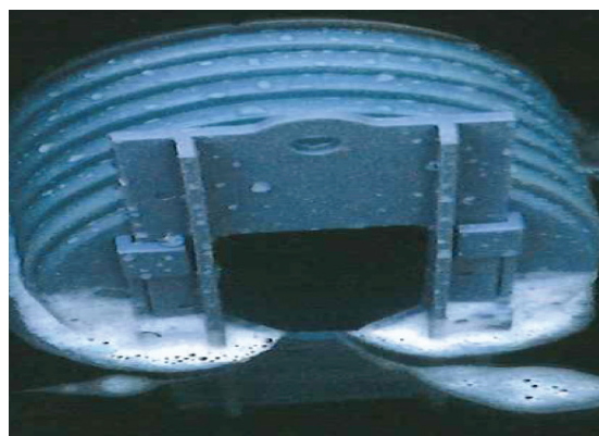
Närbild på skibord i drift. Luckan kan skjutas upp och ner med en stång som hakas fast i hålet i övre delen.
